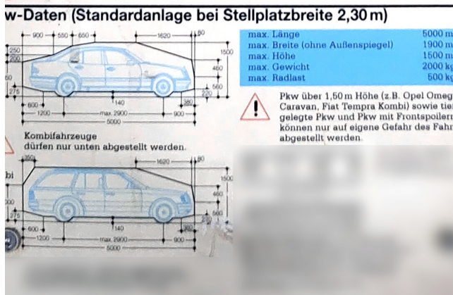
Abmessungen Duplex
